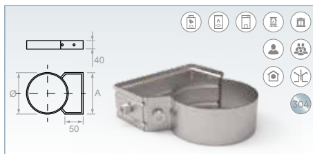
Soporte Mural (Acero Inox 304)
