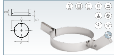
Abrazadera descenso (Acero Inox 304)
