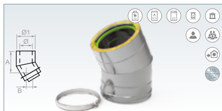
Codo 30° (Inox 316-Interior / Inox 304-Exterior)
