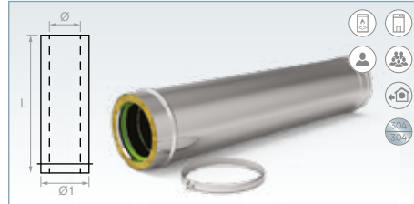
tubo Macho - Hembra (Inox 304-Interior y Exterior)
