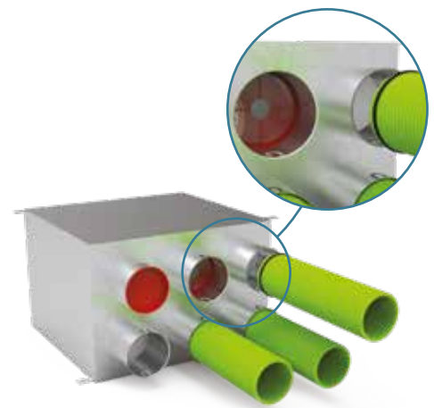
Caja de distribución con tapón, regulador de aire y tubo con junta
