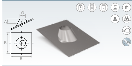
Teja inclinada 30° (Acero Inox 304)
