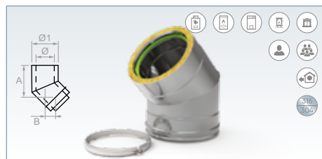
Codo 45° (Inox 316-Interior / Inox 304-Exterior)
