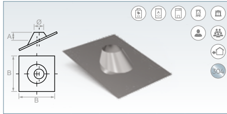
Teja inclinada 30° (Inox 304)
