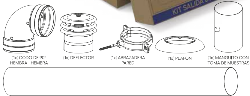
(1x) TUBO DE 1000 MM MACHO - MACHO
