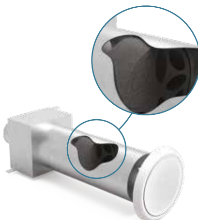
Salida horizontal con regulador de caudal y válvula de ventilación
