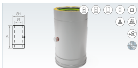
Módulo toma muestra (Inox 316-Interior / Inox 304-Exterior)
