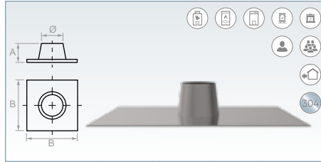
Teja plana (Acero Inox 304)
