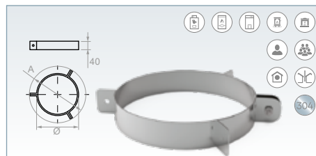
Abrazadera vientos (Inox 304)
