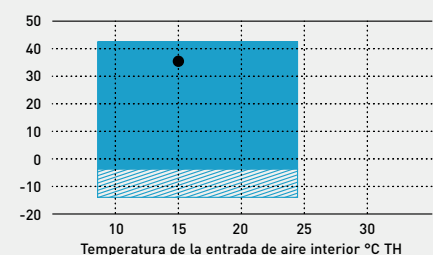
Rango de temperatura para una bodega. En refrigeración. Temperatura de la entrada de aire exterior °C TS.
