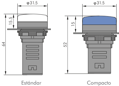
Dimensiones
