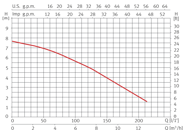
Curva de funcionamiento a 3450 rpm
